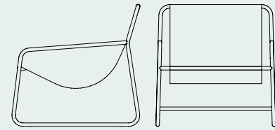
CB3502-E | 73x80 H77,5 HS32 HB50 cm
