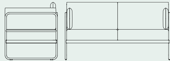
CB3503-2P E | 146x73 H80,5 HS42,5 HB66 cm
